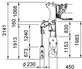
35tonフック
