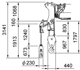
22tonフック
